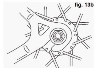
Angeschraubtes Hinterrad in den Dropouts
